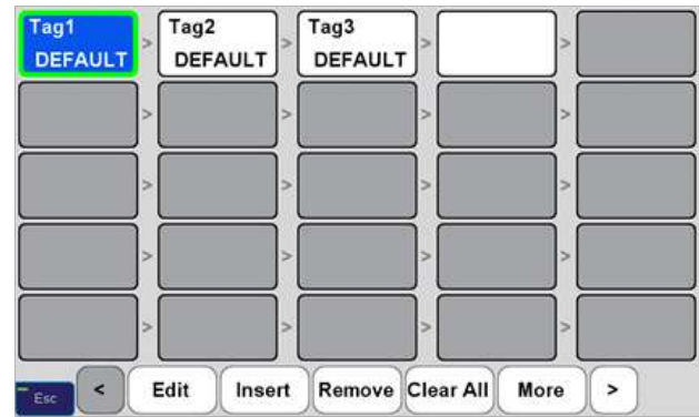
Рисунок 26. Вставка тегов
