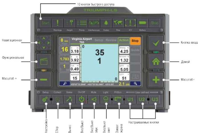
Рисунок 4. Кнопки
