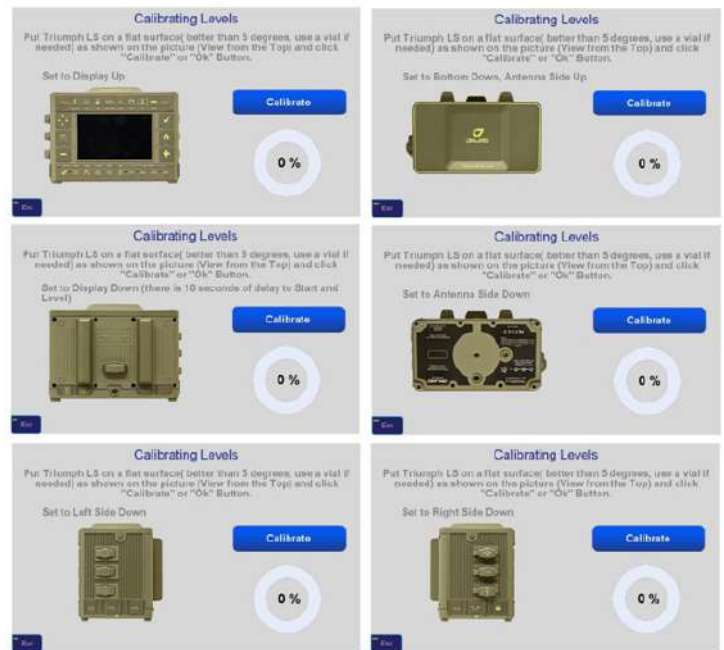
Рисунок 13. Калибровка уровней
