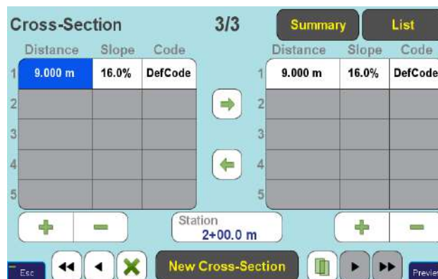
Рисунок 80. Экран Секции
