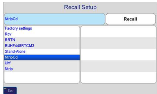
Рисунок 27. Список профилей
