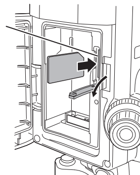
Гнездо SIM-карты
