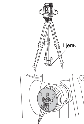
Винты точной регулировки
