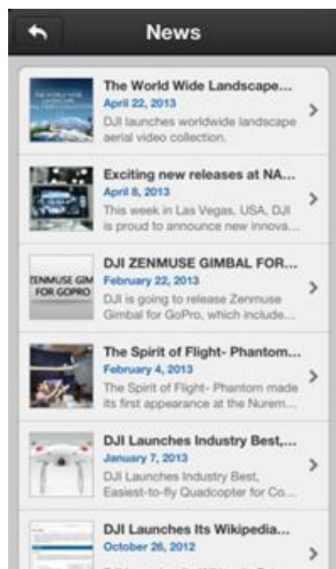
Список новостей
