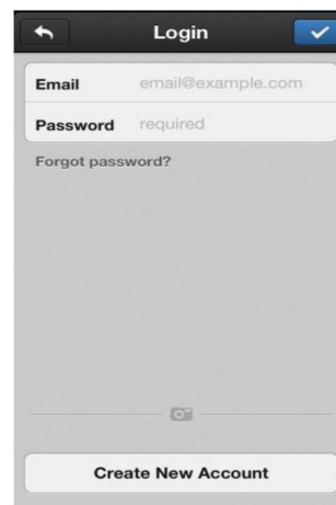
Страница входа
